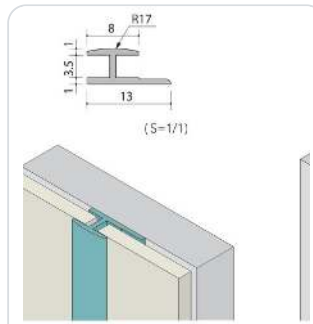
Type-A · ตัวต่อกลาง (Divider) MN-ZK-1A · ปิดรอยต่อระหว่างแผ่นให้เรียบร้อย
