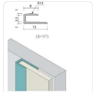
Type-B · ตัวจบขอบ (End cap) MN-ZK-1B · ปิดขอบแผ่นด้านที่ไม่ชนผนัง
