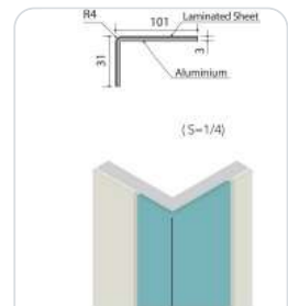
Type-L MN-ZKL · มุมเขี้ยวเล็ก
