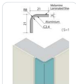
Standard Type MN-ZKH / ZKN · มุมฉากมาตรฐาน
