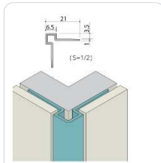
Type-D · มุมใน (Internal corner) MN-ZK-1D (สีเงินเท่านั้น) · สำหรับเข้ามุมในของผนัง
