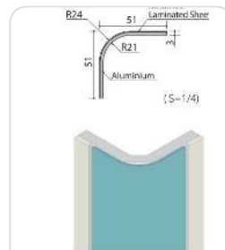
Type-G MN-ZKG · มุมโค้ง R24
