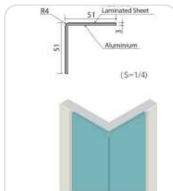
Type-J MN-ZKJ · มุมโค้ง R8
