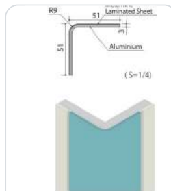
Type-F MN-ZKF · มุมโค้งหนา
