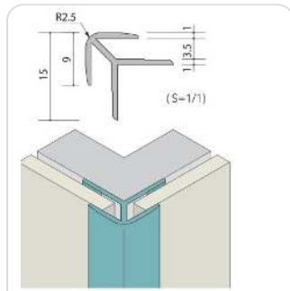
Type-C · มุมนอก (External corner) MN-ZK-1C / ZKC-1C · 2 ชั้น/ชุด ยาว 3,075 มม. สำหรับเข้ามุมนอก 90°
